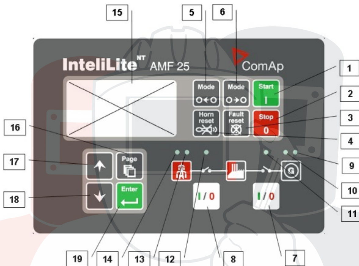
КНОПКИ УПРАВЛЕНИЯ ГЕНЕРАТОРНОЙ УСТАНОВКОЙ
